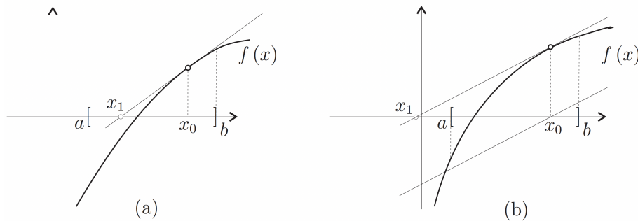
Figura 5.1: Mètode de Newton-Raphson
