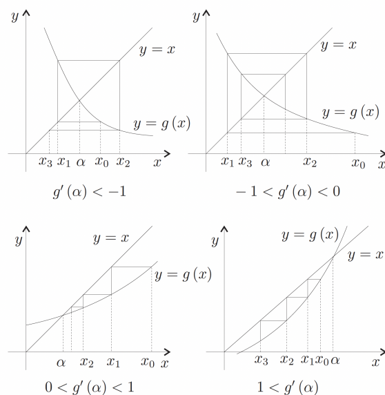
Figura 5.2: Tipus de comportament de x_{k+1} = \varphi(x_k) al voltant d'un punt fix.
